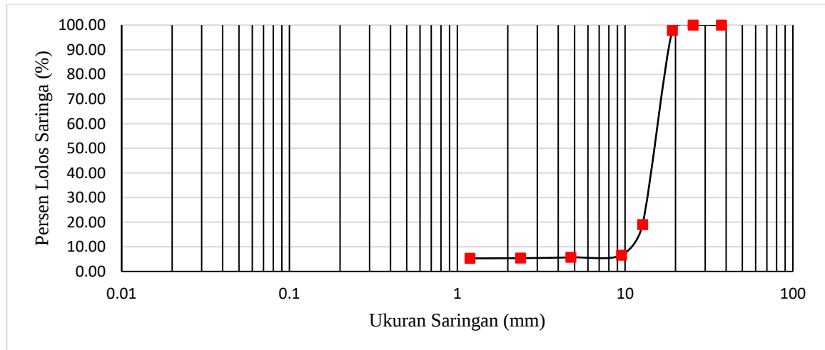
Gambar 4 Kurva Kategori 20 mm Agregat Kasar Cinangsih Sumber : Dokumen Pribadi
