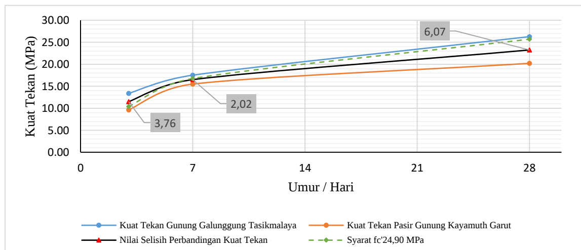
Gambar 5 Grafik Perbandingan Kuat Tekan Beton
