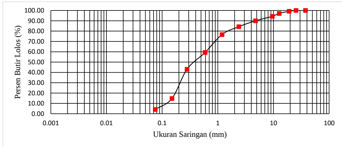
Gambar 2 Kurva Gradasi Agregat Halus Gunung Galunggung Tasikmalaya
