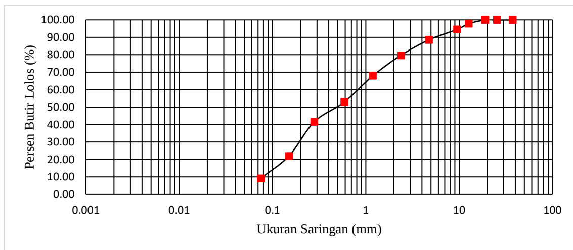
Gambar 3 Kurva Gradasi Agregat Halus Gunung Kayamuth Garut
