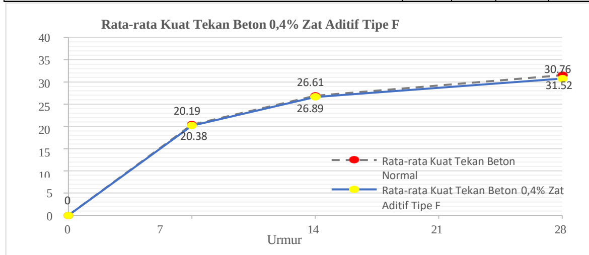
Gambar 7 Grafik Hasil Pengujian Kuat Tekan Beton 0,4% Zat Aditif Tipe
