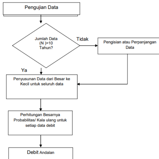
Gambar 1. Tahapan Analisa Debit Sungai Menggunakan Lengkung Kekerapan Untuk Data Menerus Sumber: Modul Perhitungan Hidrologi Pelatihan Perencanaan Bendungan Tingkat Dasar Kementerian PUPR 2017
