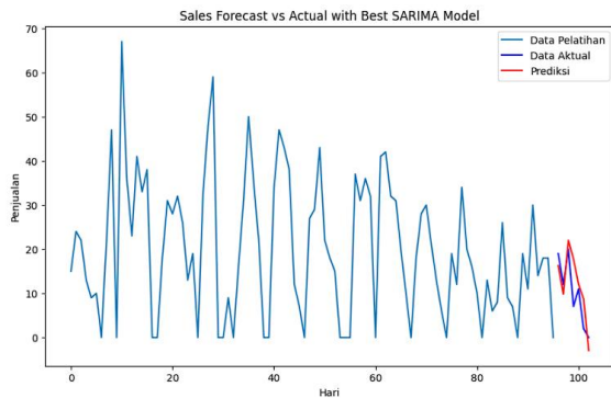
Gambar 9. Grafik Data Awal, Aktual Dan Prediksi
