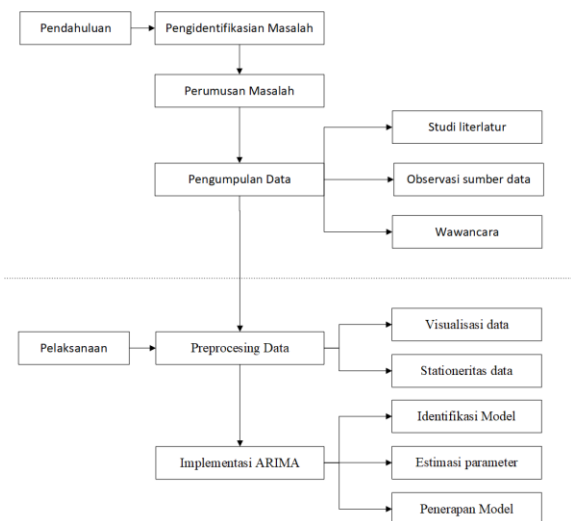
Gambar 2. Tahap Penelitian
