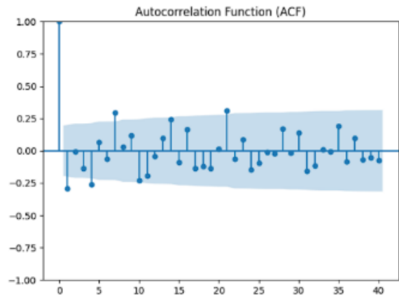
Gambar 5. Grafik ACF
