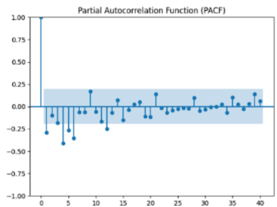
Gambar 6. Grafik PACF
