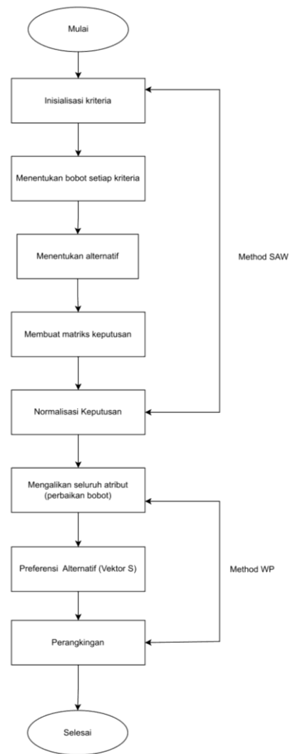
Gambar 3. Tahapan impementasi program
