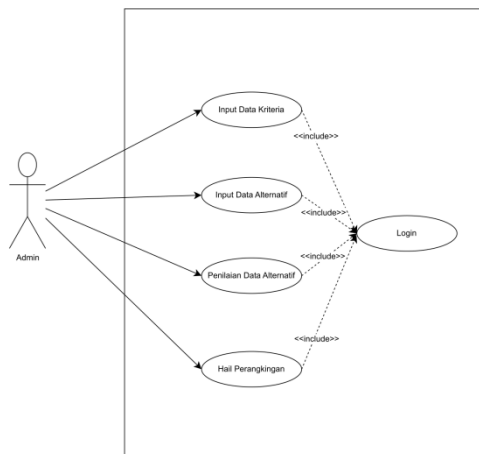
Gambar 4. Rancangan Use Case
