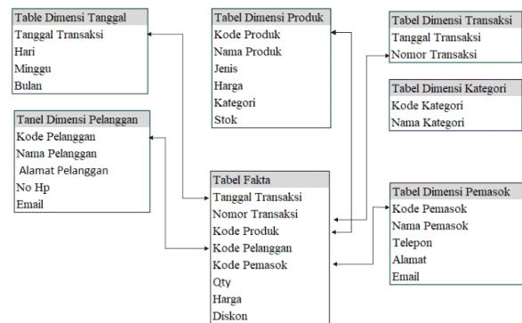
Gambar 3. Skema snowflake
