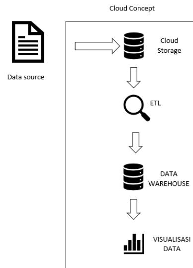
Gambar. 2 Cloud Konsep
