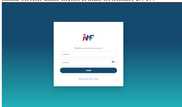
Gambar 6. Halaman Login
