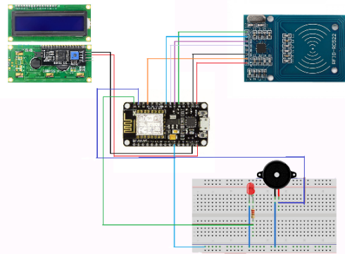
Gambar 5. Rangkaian Sistem
